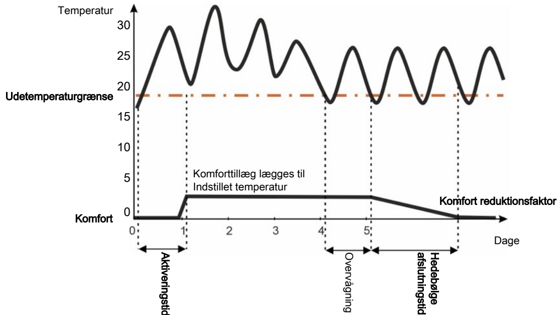
Figur 5: Hedebølge-komfort
