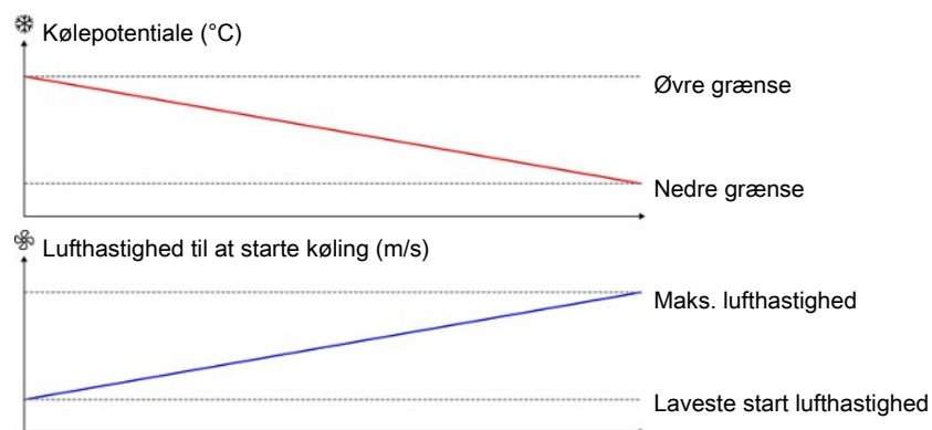
Figur 31: I områder med lav udefugt og et stort kølepotentiale, kan kølingen starte ved en lavere lufthastighed. Omvendt vil man i områder med lavt kølepotentiale vente så længe som muligt med at starte kølingen, så den starter ved maksimum lufthastighed.
