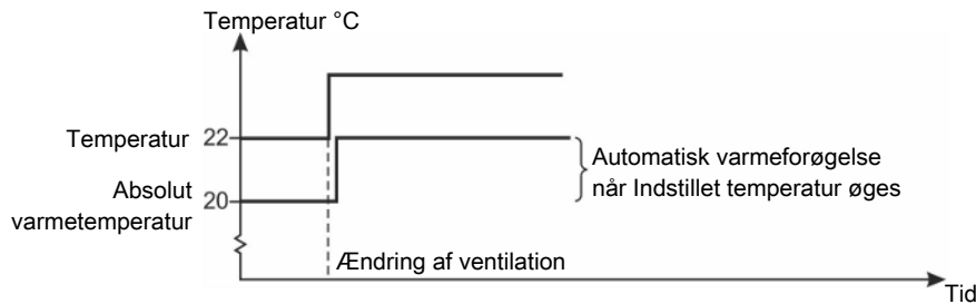
Figur 34: Varmetilsætning
