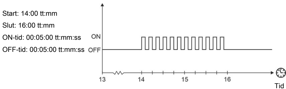
Figur 22: Døgnursregulering
