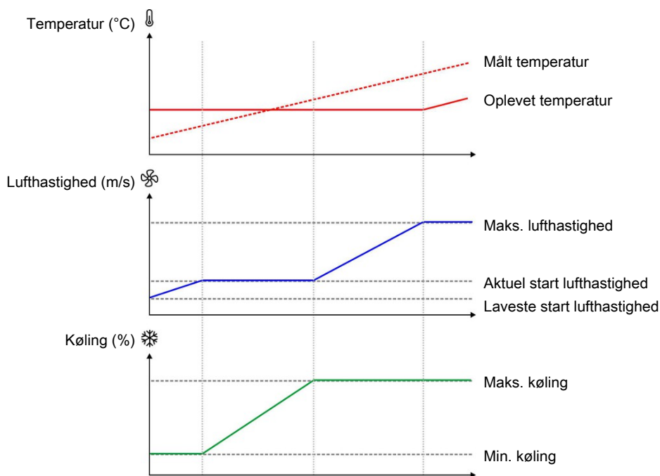
Figur 32: Kølingen starter allerede ved lav lufthastighed for at holde den ønskede indetemperatur. Når kølingen ikke kan holde temperaturen, øges lufthastigheden igen.
