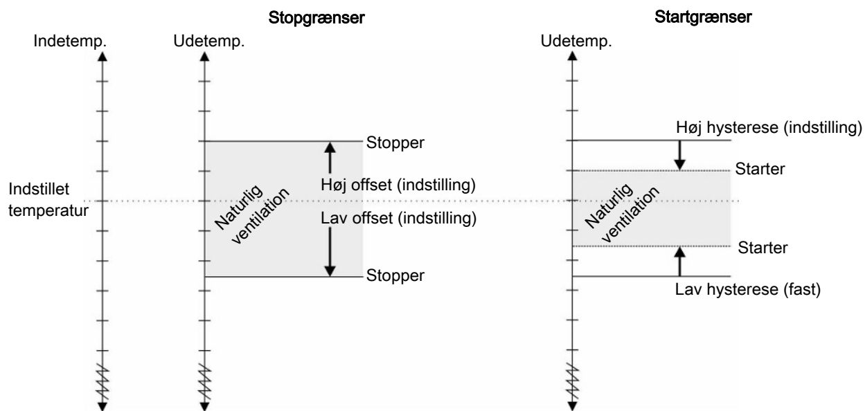
Figur 20: Start og stop i forhold til udetemperatur. Temperaturgrænserne indstilles som offset i forhold til indstillet temperatur.
